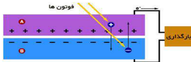
(A) -سيليكون نوع N و (B) سيليكون نوع P عملكرد سلول فوتوولتايي
